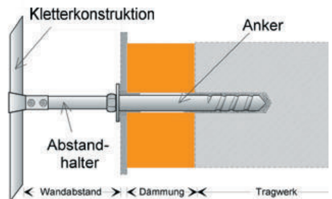
Schema Wärmedämmverbundsystem (WDVS): Sonderlösung nicht inkludiert - gegen Aufpreis optional möglich
