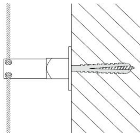
Schema Standardlösung Massivmauerwerk (inkludiert im Paket)
