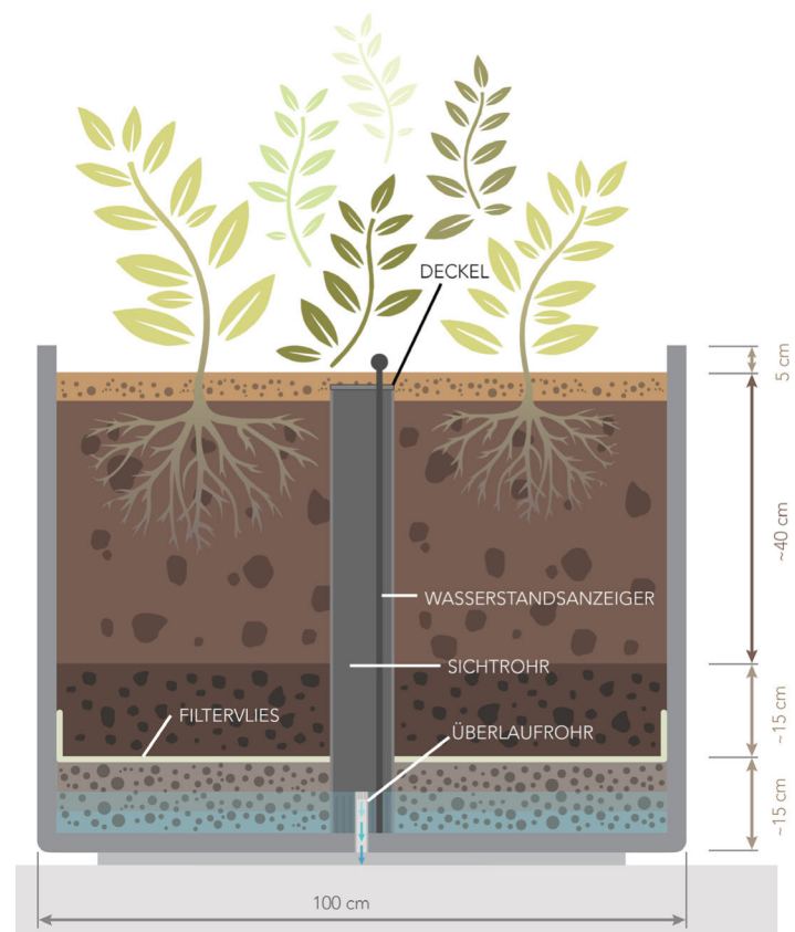
Schnitt von vorne © GRÜNSTATTTGRAU
