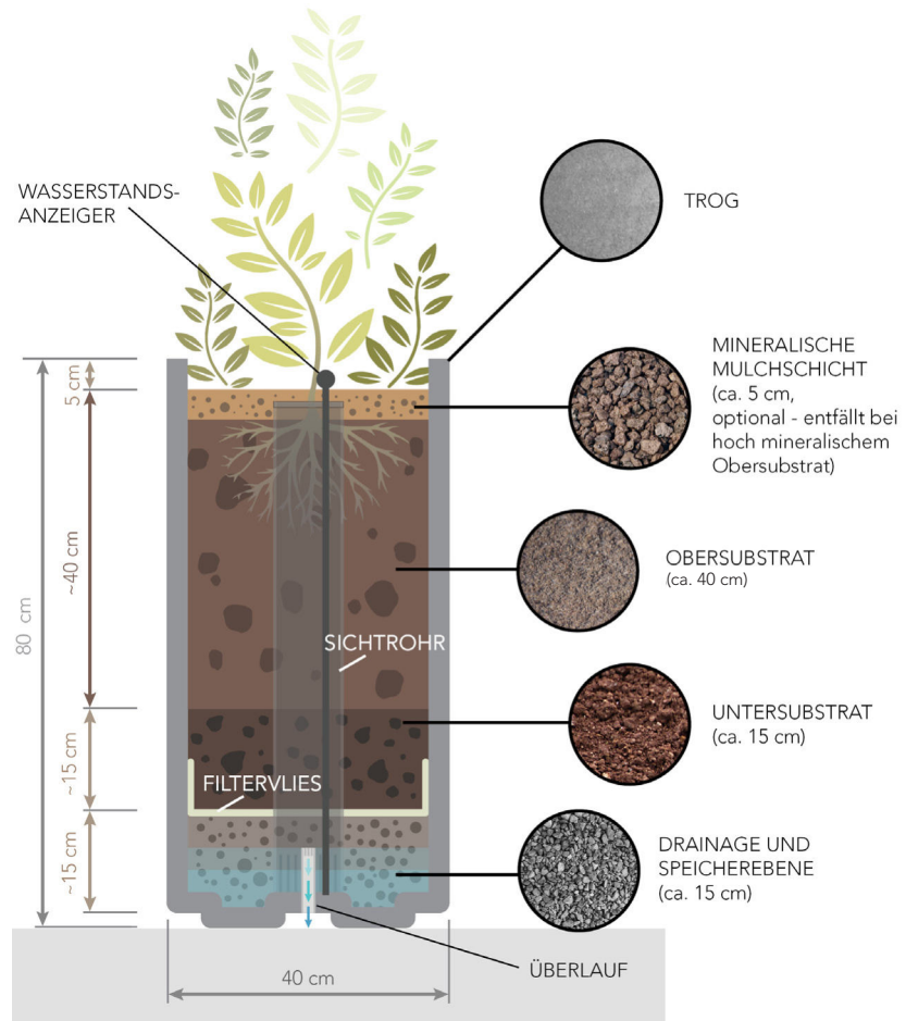
Schnitt seitlich © GRÜNSTATTTGRAU
